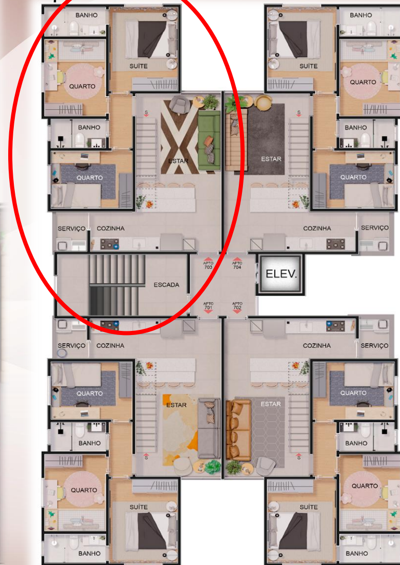
PLANTA 7º PAVIMENTO - COBERTURA
