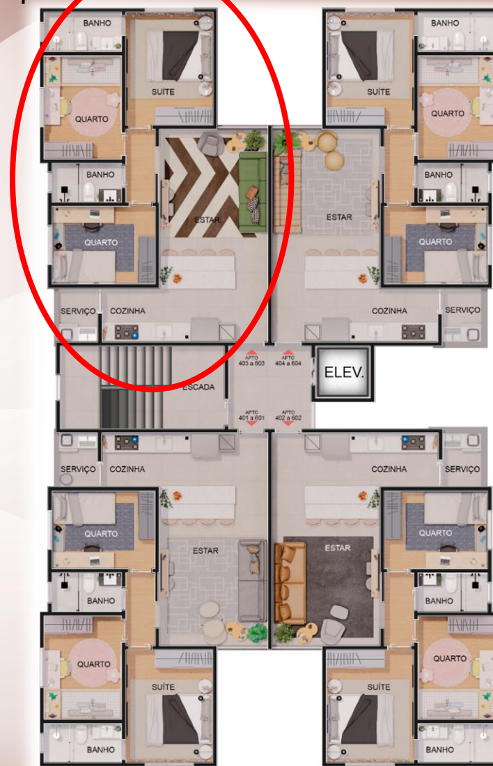
PLANTA 4º a 6º PAVIMENTO - APARTAMENTOS TIPO
